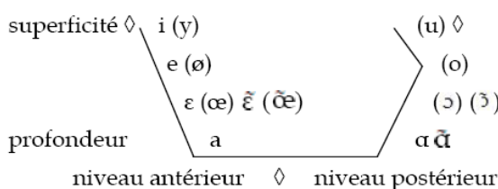
Fig. 2 : Les voyelles en français
