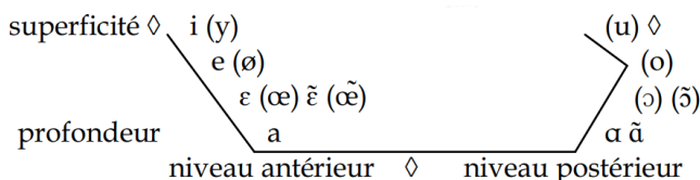
Sch. 1: Sistemul vocalic al limbii franceze
